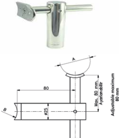
► KZNİ-D7500-3
