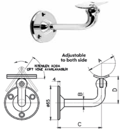
► KZNİ-D7500-6
