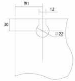
► KZNI-8600C-1 SÜRME KAPI TEKERLEĞİ Cam Delik Ölçüleri
