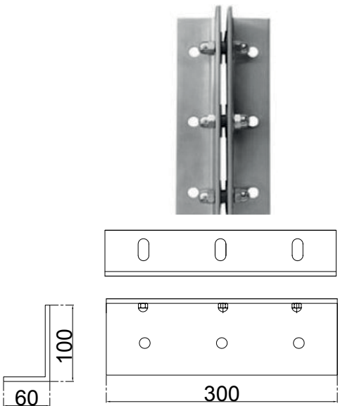
► KZNi-SC-03
