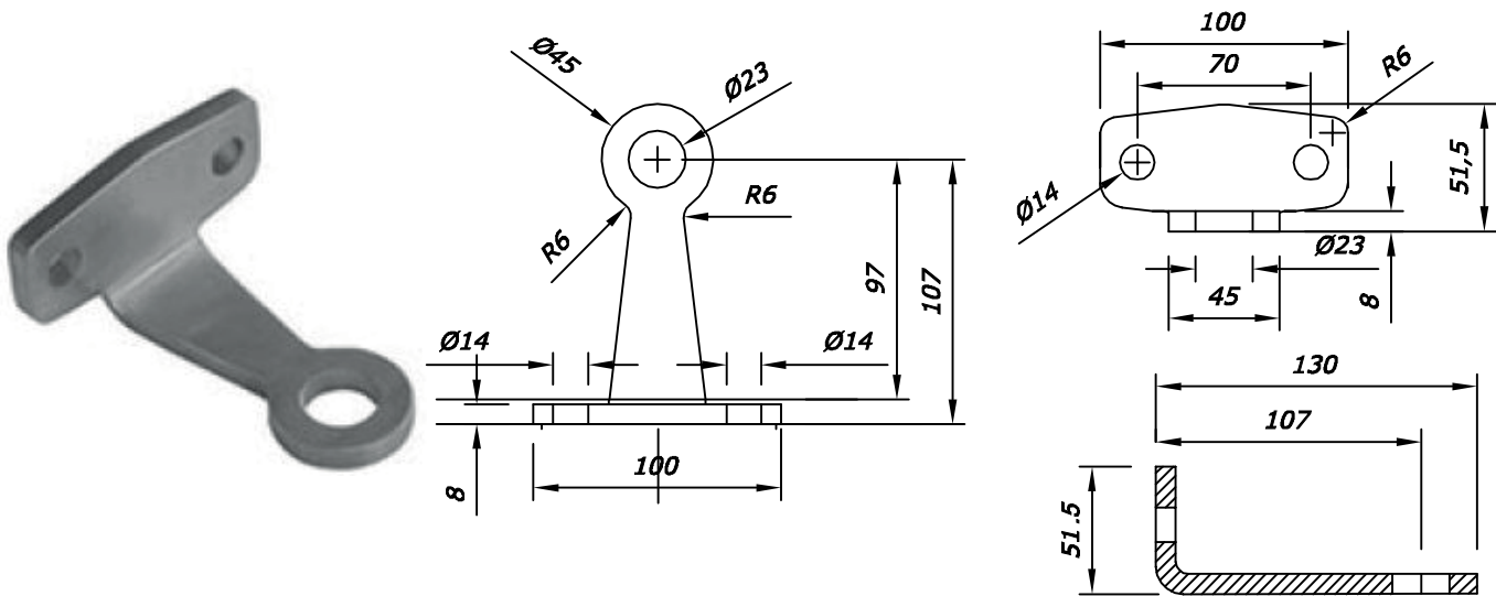
► KZNi-SC-02
