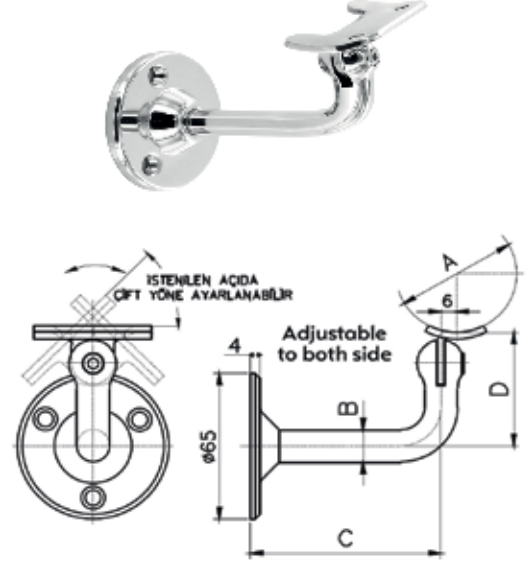
► KZNİ-D7500-5
