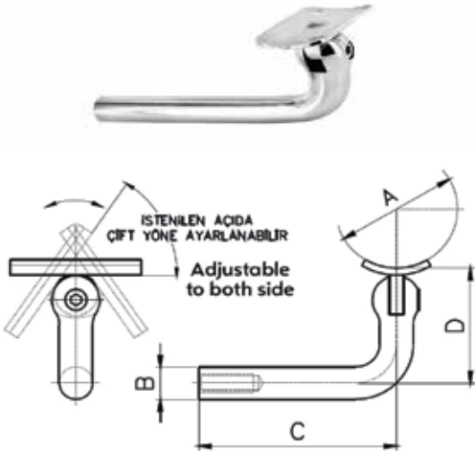
► KZNİ-D7500-3
