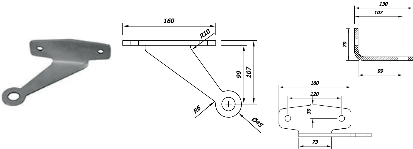
► KZNi-SC-02
