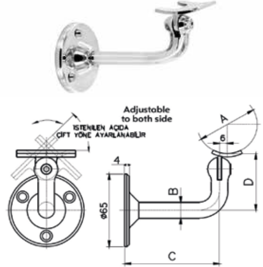
► KZNİ-D7500-6
