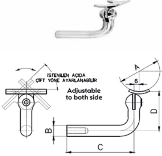
► KZNİ-D7500-2
